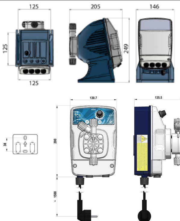
Fig. 1 - Dimensões em mm. Placa para a fixação de parede.
