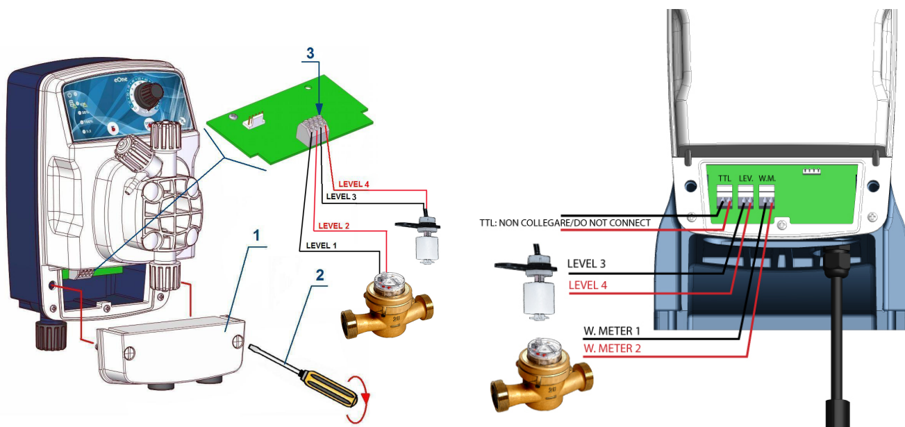
Fig. 9 – Indicações para o cabeamento da sonda de nível e contador
