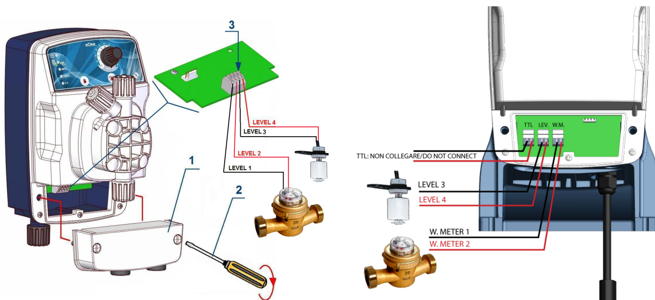
Fig. 9 – Indications pour le câblage de la sonde de niveau et compteur
