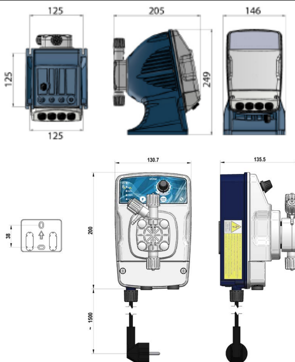
Fig. 1 - Dimensioni in mm. Placca per il fissaggio a parete.
