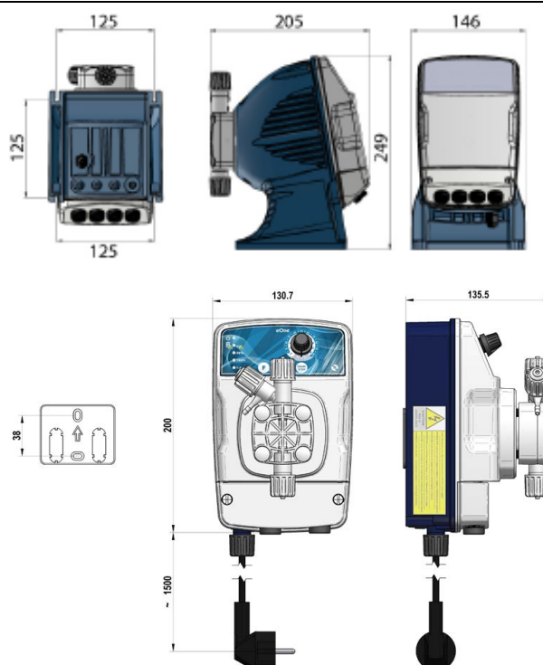
Fig. 1 - Dimensions en mm. Plaque pour la fixation murale.
