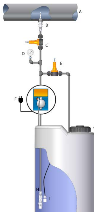
Fig. 6 – Instalación típica
