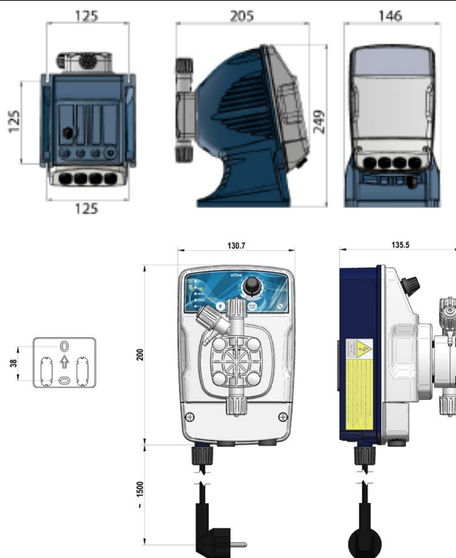
Fig. 1 - Dimensiones en mm. Placa para la fijación en pared.
