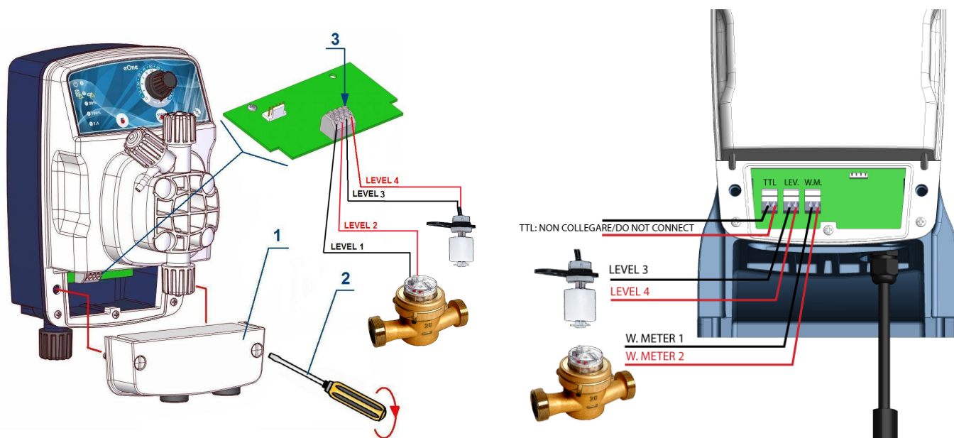
Fig. 9 – Indicazioni per il cablaggio della sonda di livello e contatore
