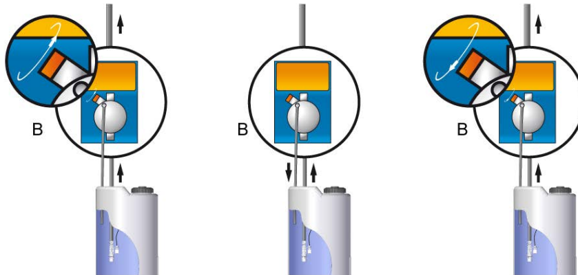
Fig.5 – Actionnement vidange par amorçage
