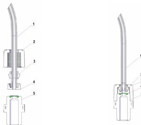
Fig.4 – Ligação hidráulica
