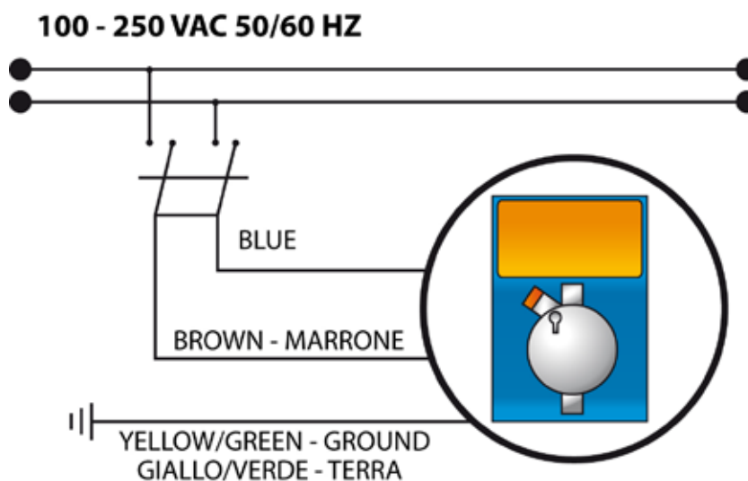
Fig.3 - Branchement électrique
