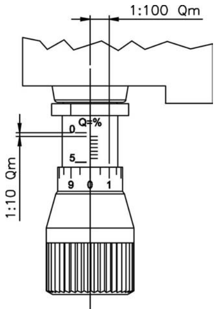
Fig. 16 - pomo de regulación
