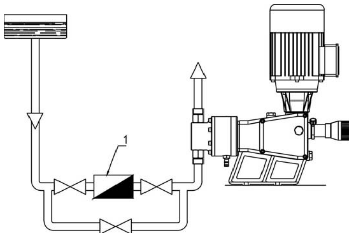
Fig. 12 – Layout para dosagem de líquidos com impurezas
