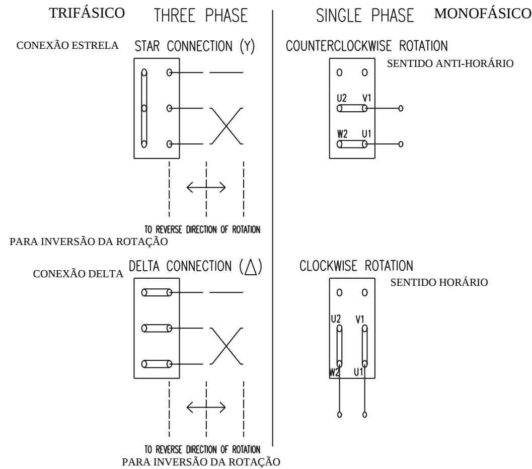
Fig. 17 - Conexão à rede eléctrica
