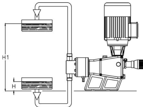
Fig. 11 – instalação / sucção elevada
