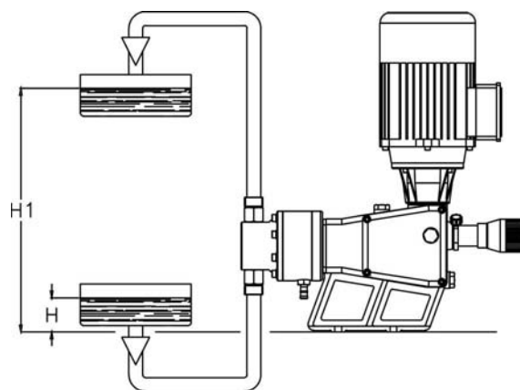
Fig. 8 – installation sur battant
