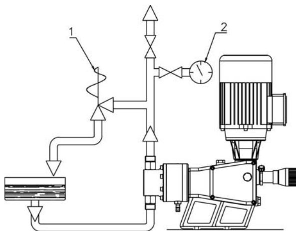
Fig. 4 - dispositifs de sécurité
