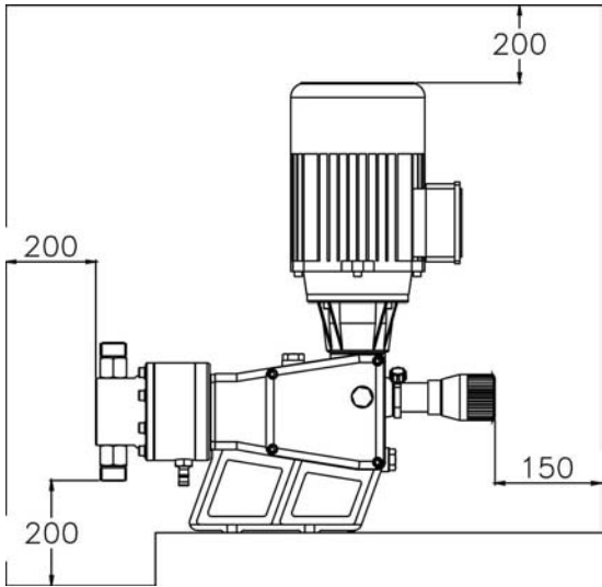
Fig. 6 – Espaço de trabalho mínimo (mm)
