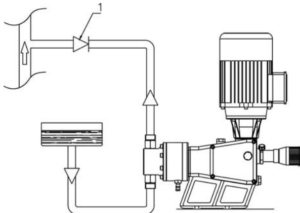
Fig. 13 – instalación con válvula de inyección impelente
