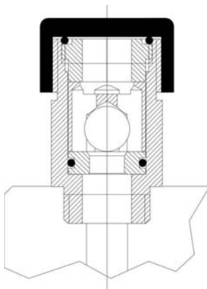
Fig. 14 – Tampas protectoras
