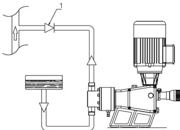
Fig. 13 – Válvula de injeção instalada na tubagem de descarga
