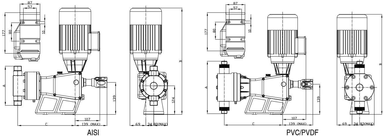
Fig. 2 Dimensions d'encombrement (mm)
