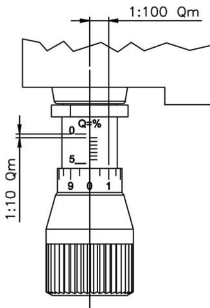
Fig. 16 – Ajuste micrométrico
