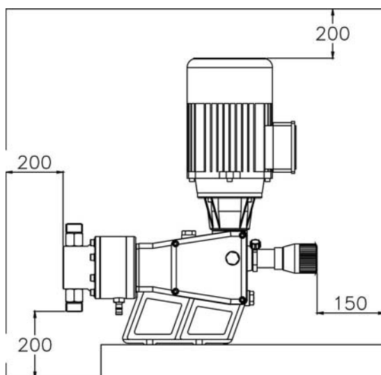
Fig. 3 - distances minimum en mm
