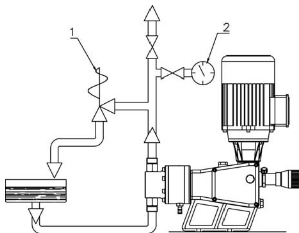
Fig. 7 – Válvula de alívio
