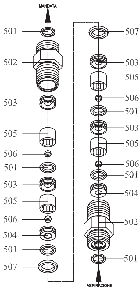
VÁLVULA DUPLA ESFERA
