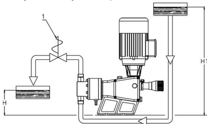
Fig. 10 – Instalação com sucção afogada
