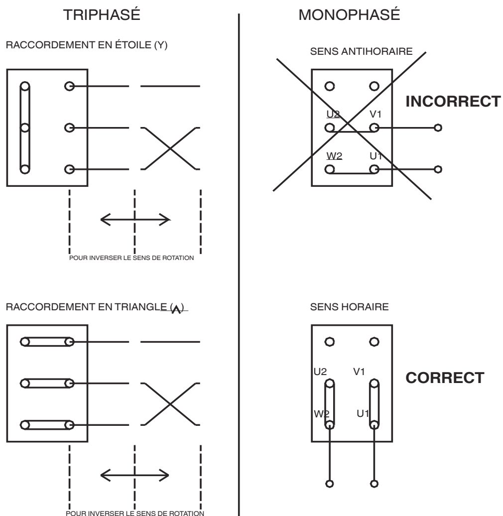
Fig. 14 - Schéma de raccordement au réseau électrique
