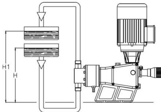
Fig. 9 - installazione ideale
