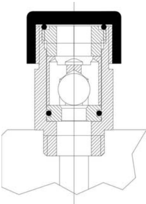
Fig. 14 - tapón de protección
