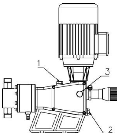
Fig. 15 – Posições das tampas de óleo
