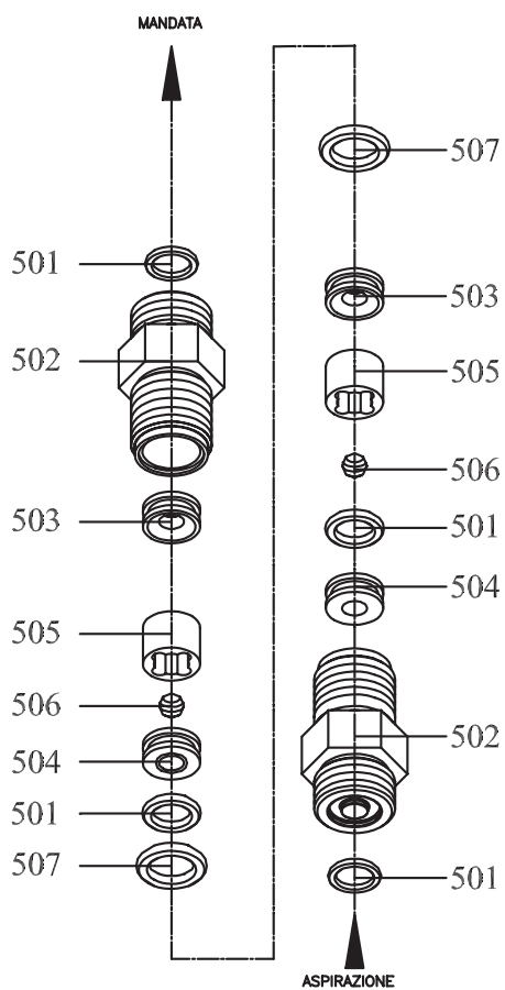
VÁLVULA ESFERA SIMPLES
